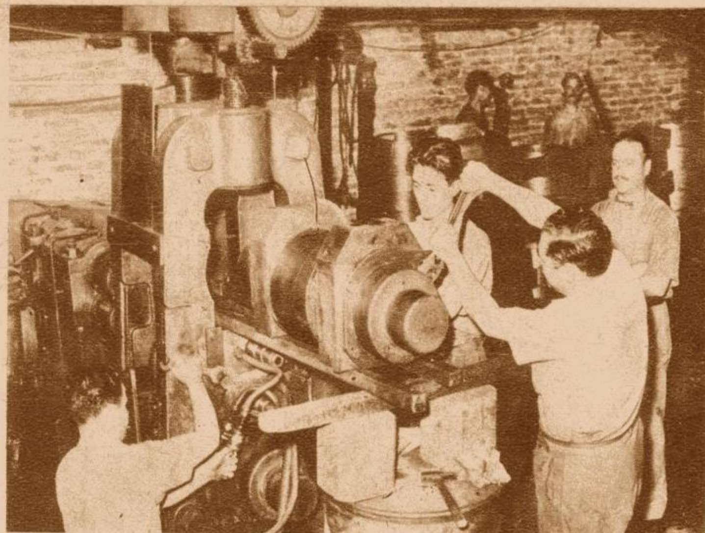
CAMBIO DE CILINDROS EN LAMINACION EN FRIO. Para que los materiales sean perfectos y no existan diferencias en sus espesores, es necesario el cambio de cilindros en forma periódica. Esta fotografía demuestra el instante que se procede a ello.
