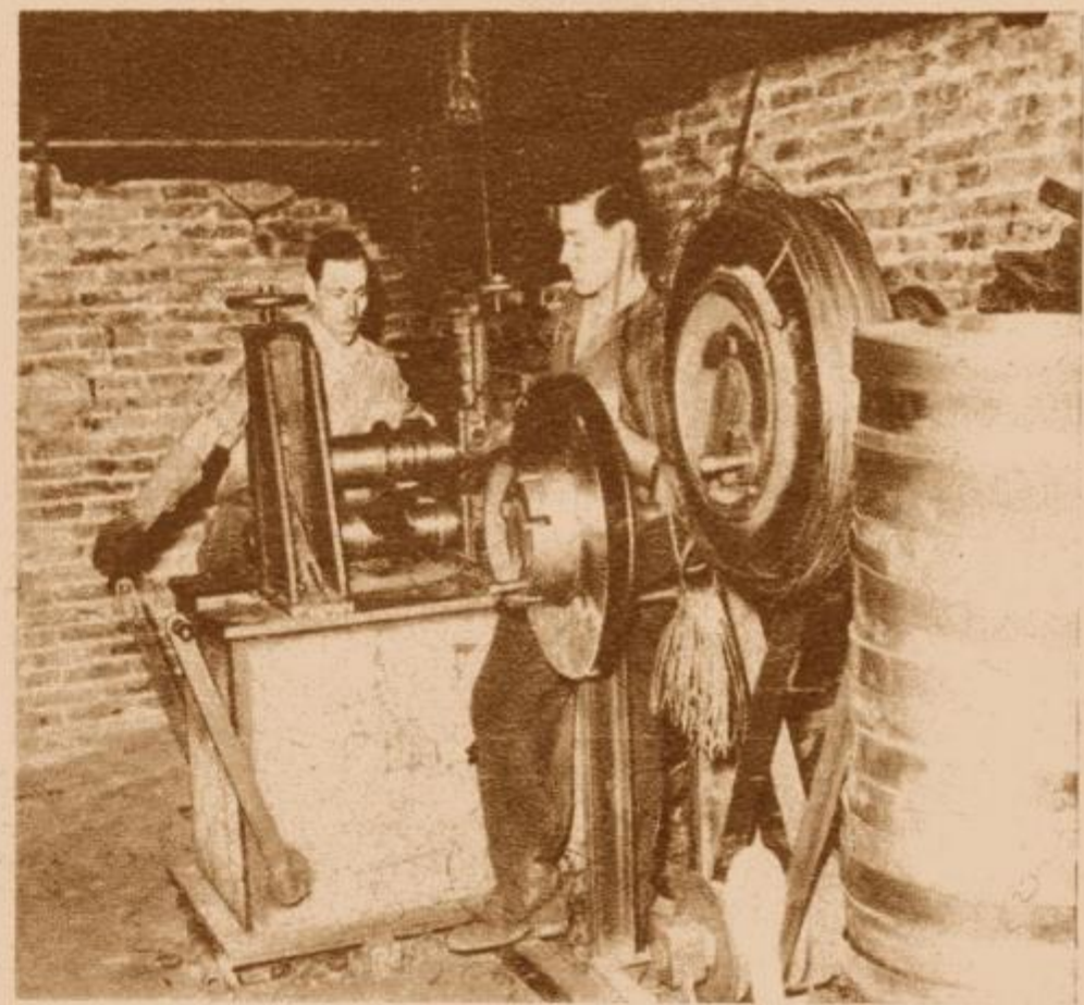
CORTANDO EL FLEJE. Una vez laminados los mismos, son cortados de acuerdo a las necesidades del consumidor. Esta máquina ha sido construída en el mismo taller, siendo su resultado magnífico y de gran rendimiento comparada a otras similares fabricadas en los más importantes centros industriales del mundo.
