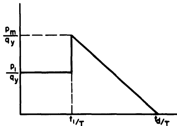
(d) Triangular Pulse With Rectangular Precursor
