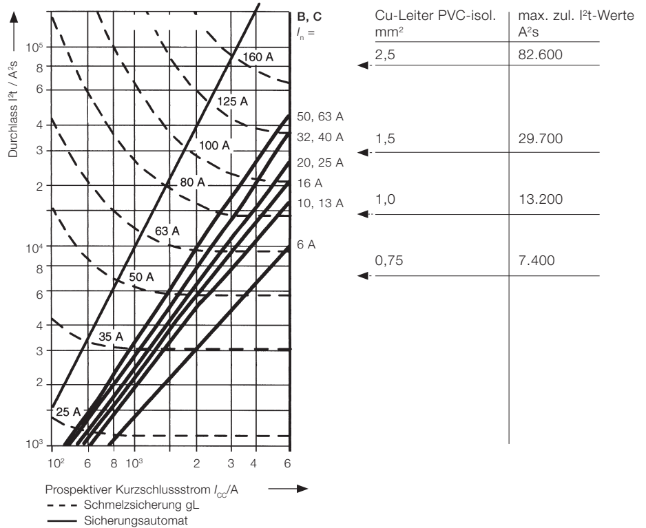
Abb. 2 Durchlassenergie I^2t
