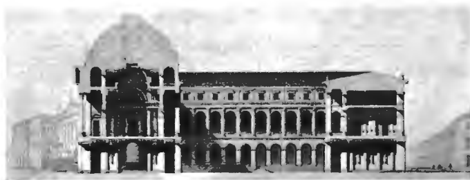
Проектъ зданія Сената (въ разрѣзѣ) архит. Жако.
