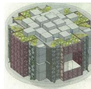
図2 与圧部内の荷物の搭載性向上
