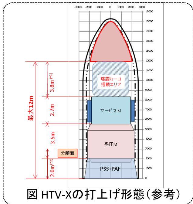
HTV-X (日本)
