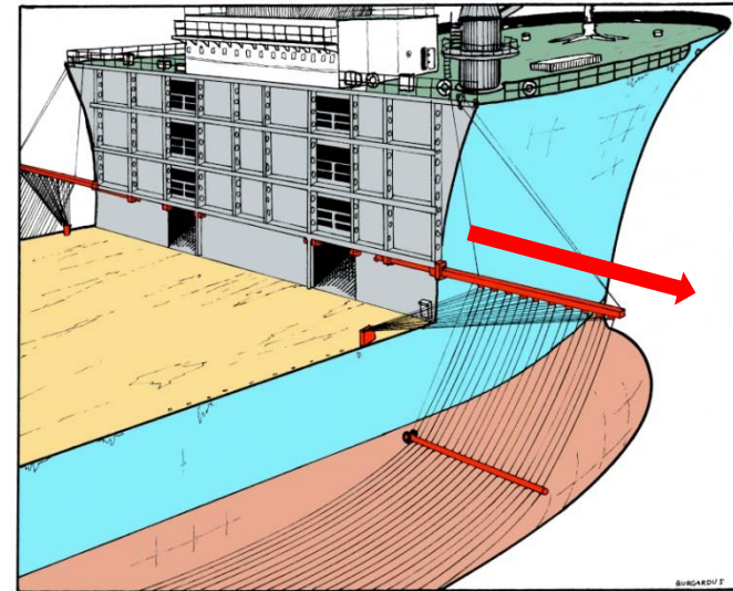
Slidingboom
