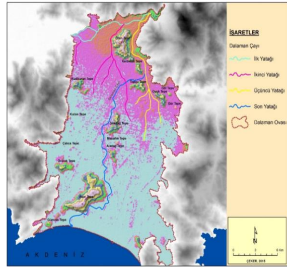
Şekil 1: Dalaman Çayı'nın Yatak Değişimleri ve Dalaman Ovası'nın Oluşumu
