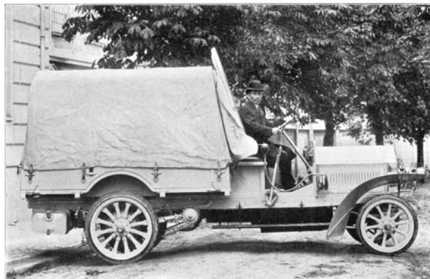
Automobil RAF – lehký užitkový automobil – nosnost do 1 500 kg, rok výroby 1912. Materiály zpracovány ve spolupráci s Národním technickým muzeem v Praze, letos uplyne 100 let od jeho založení.
