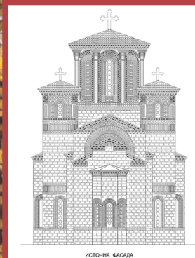
Источна фасада – црква East facade – church
