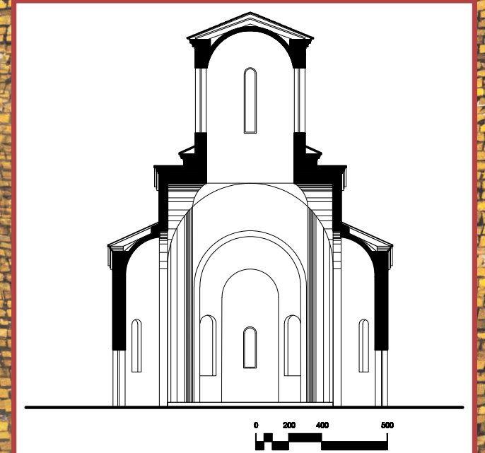
Пресек – црква – попречен Cross – section – church
