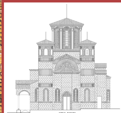
Јужна фасада – црква South facade – church
