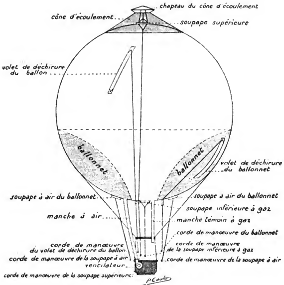
Le ballon le Djinn (fig. schematique)
