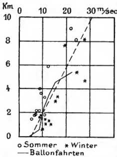
Fig. 7. — Wolkenhöhe und -Geschwindigkeit.
