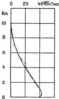
Fig. 10. — Stärke der Dampfströmung.
