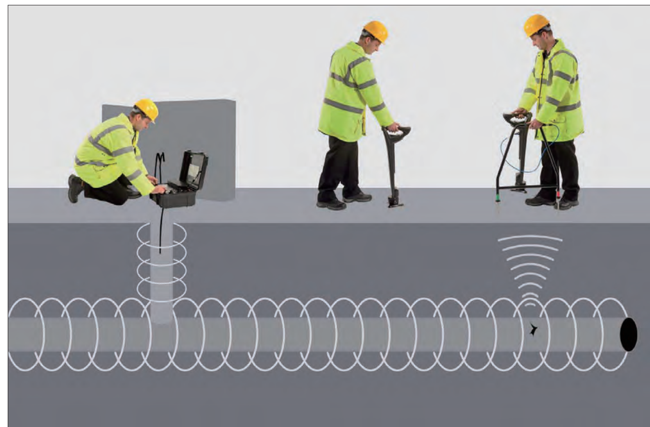
外检测之ACVG检测示意图
