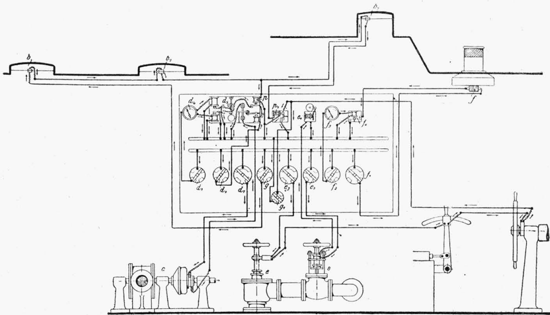
18. ábra. Kapcsolási vázlat a merülőhajó jelzőberendezéséről.
