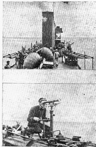
20. ábra. Torpedó lanszirozó elhelyezése egy amerikai torpedó-üldözőn (fenn), célzó és beállító készülék kezelése (lenn).
