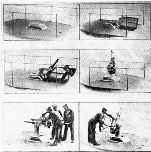
22. ábra. A legújabb Krupp-féle gyorstüzelő ágyu elhelyezése és kezelése.
