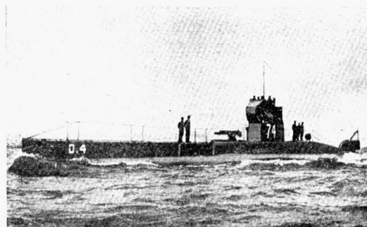
23. ábra. A gyorstüzelő ágyu elhelyezése egy nagy típusú angol merülőhajón.
