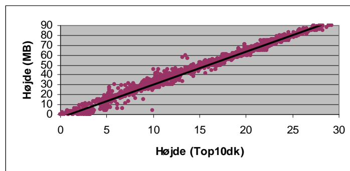
Figur 9: Relation mellem højde på Det Høje Målebordsblad (fod) og Top10dk (meter). Tendenslinie; y = 3,3314x - 2,9416 . R^2 ; 0,9857.
