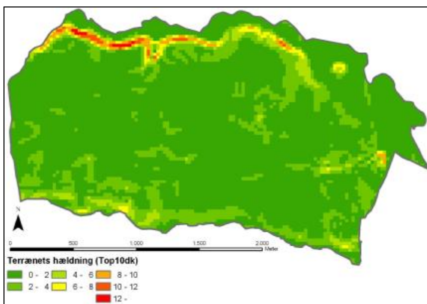
Figur 11: Hældningskort udarbejdet på grundlag af det moderne Top10dk kort.
