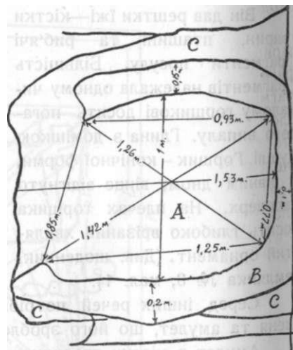
Мал. 2. План печи: А—піч. В—стінки печи. С—підмурок печи.
