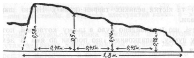
Мал. 3. Схематичний профіль печі.
