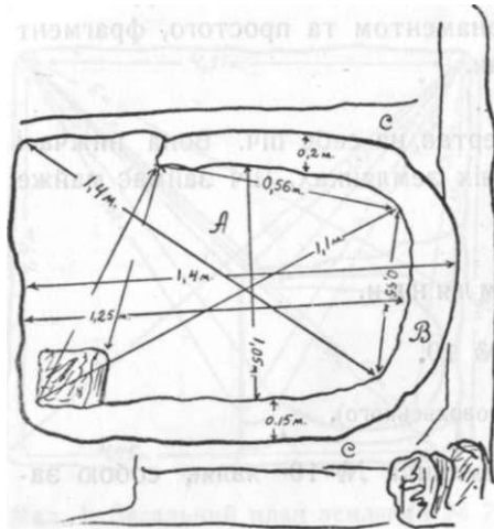
Мал. 2. План печі. А—піч. В—стінки печі. С—підмурок печі
