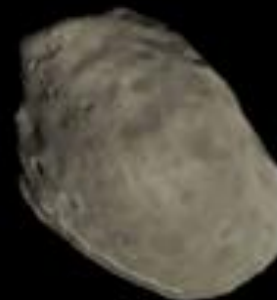
Mars Moons
