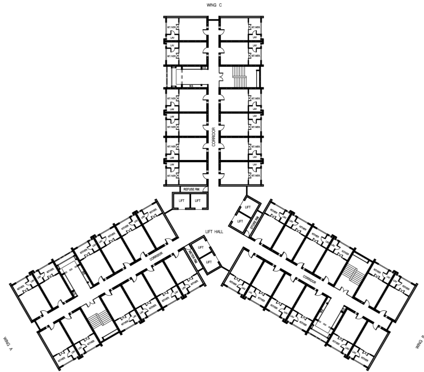
標準型大廈 Y-型 標準樓層平面圖
