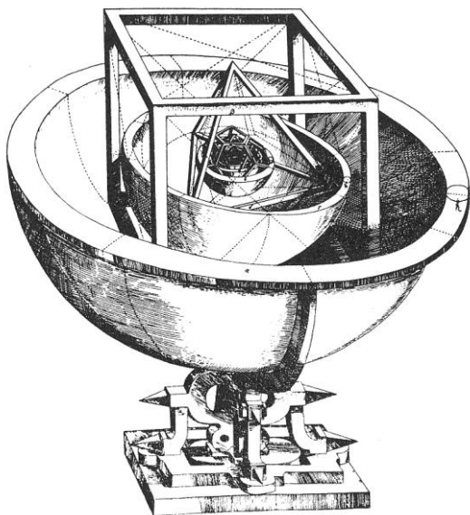
Abb. 8 Johannes Kepler, Weltmodell Sog. „Machina mundi artificialis“, 1596
