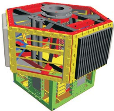
6-секторная коммутируемая 16-канальная АФАР для мобильной связной радиорелейной станции с полным азимутальным обзором
