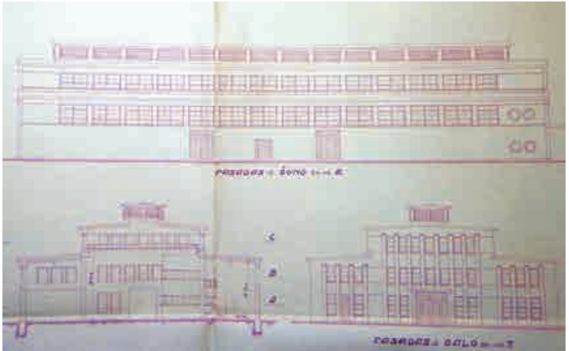
Ginklavimo valdybos civilinio tarnautojo architekto B. Elsbergo suprojektuoto Linkaičių ginklų dirbtuvių Artilerijos skyriaus pastato H fasado brėžinys.
