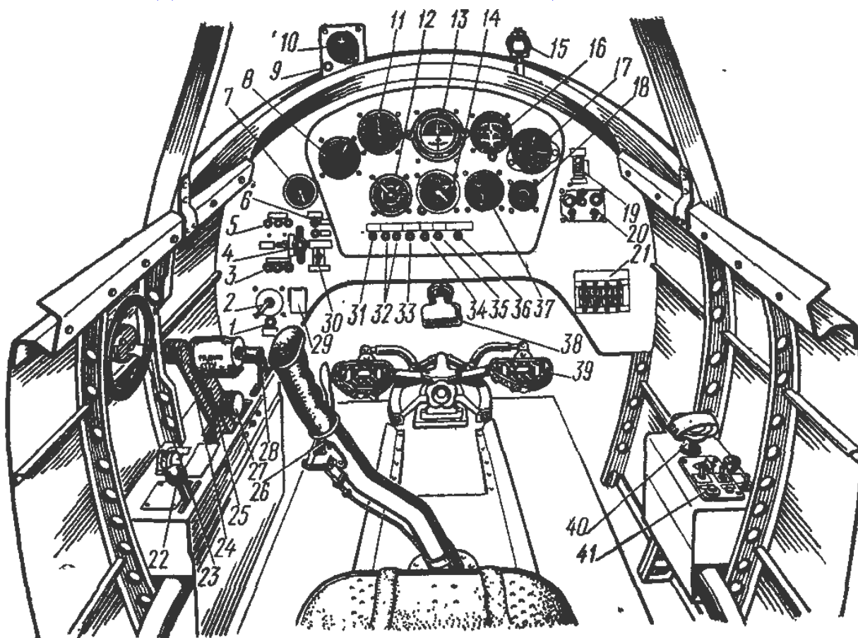
Рис. 4 Задняя кабина самолета
