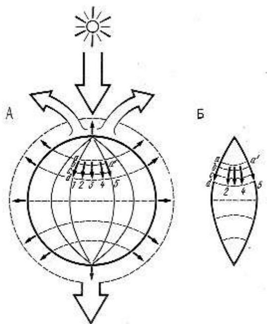
Рис. 3.6. Потoki энергии и механизм обеспечения надежности биотических систем в биосфере: 1, 2, 3... — потоки энергии через виды, а — а1... — связи между ними; А — состояние до уничтожения вида 3; Б — вид 3 исчез, проходившие через него потоки энергии идут через дублирующие виды 2 и 4
