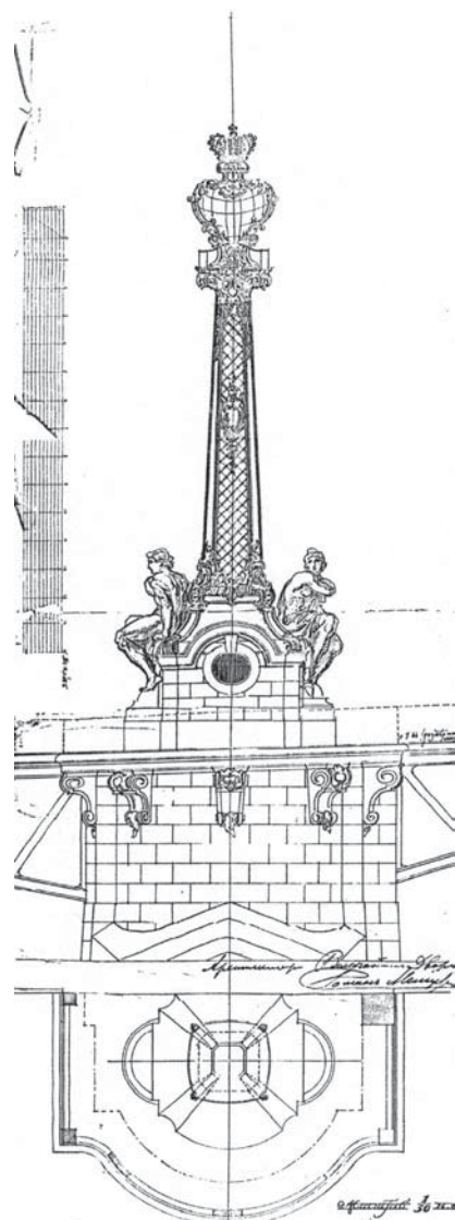
Проект фонарного столба для быков № 3 и 4 разводного пролета. Арх. Р. Ф. Мельцер. 1910 г.
