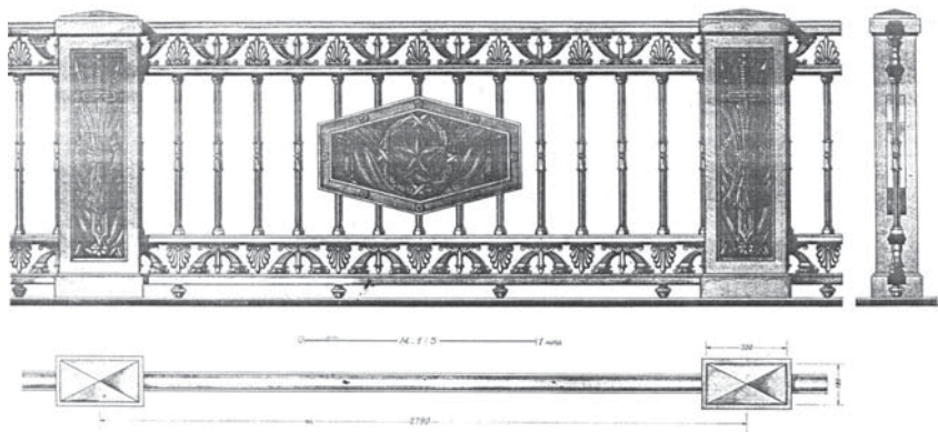
Проект чугунной решетки Дворцового моста арх. Л. А. Носкова. 1939 г. Архив «Мостотреста»
