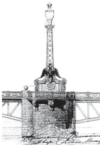
Проект упрощенного фонаря для Дворцового моста арх. Р. Ф. Мельцера. 1913 г.
