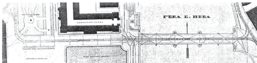
Эскизный проект внешнего вида Дворцового моста. Худ.-арх. Р. Ф. Мельцер (Зодчий. 1915. № 46)
