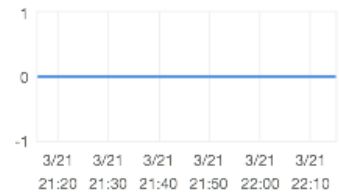
FreeStorageSpace (Megabytes)
