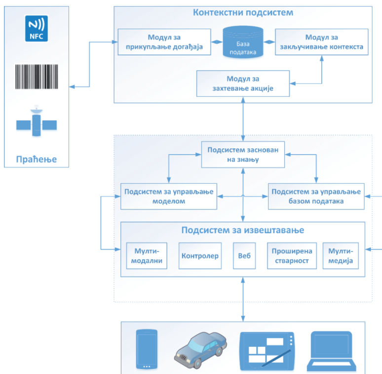
Слика 6. CONTEXT-AWARE СИСТЕМ
