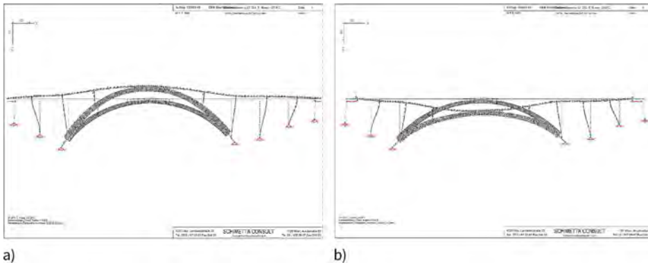
Bild 4.10 Temperaturverhalten des Überbaus bei a) Erwärmung und b) Abkühlung
