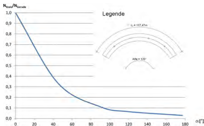
Bild 4.8 Einfluss der Krümmung auf die Normalkraft im Überbau
