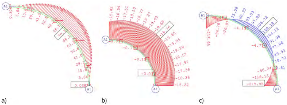
Bild 4.9 a) Verschiebungen, b) Normalkraft und c) Biegemomente eines gekrümmten integralen Tragwerks
