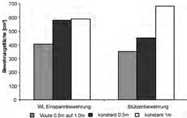
Bild 4.4 Reduzierung der Bewehrungsmengen infolge einer Voute
