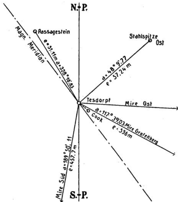
Fig. 2. Situationsplan der Miren für die erdmagnetischen Beobachtungen.
