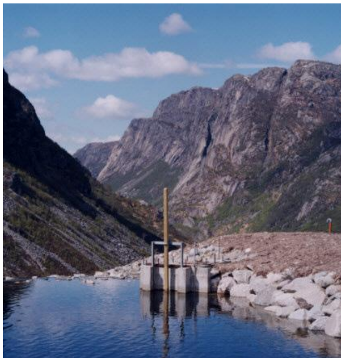
Bildet viser inntakskummen på Byrkjedal kraftverk, bygget i 1998.
