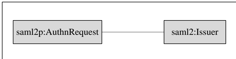
Рисунок 7 – Структура AuthnRequest
