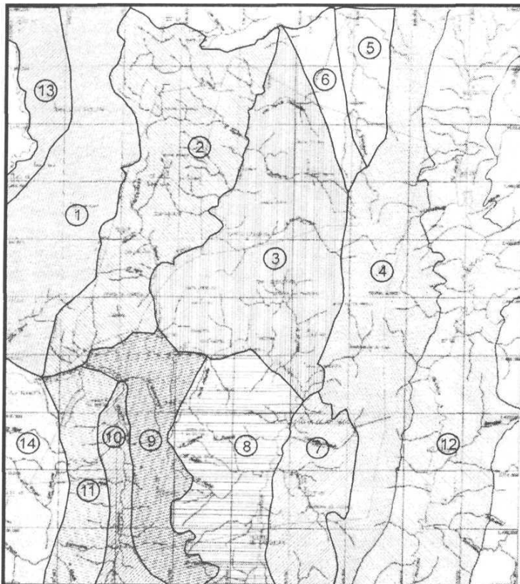
Figura 13. Regiones geomorfológicas.
