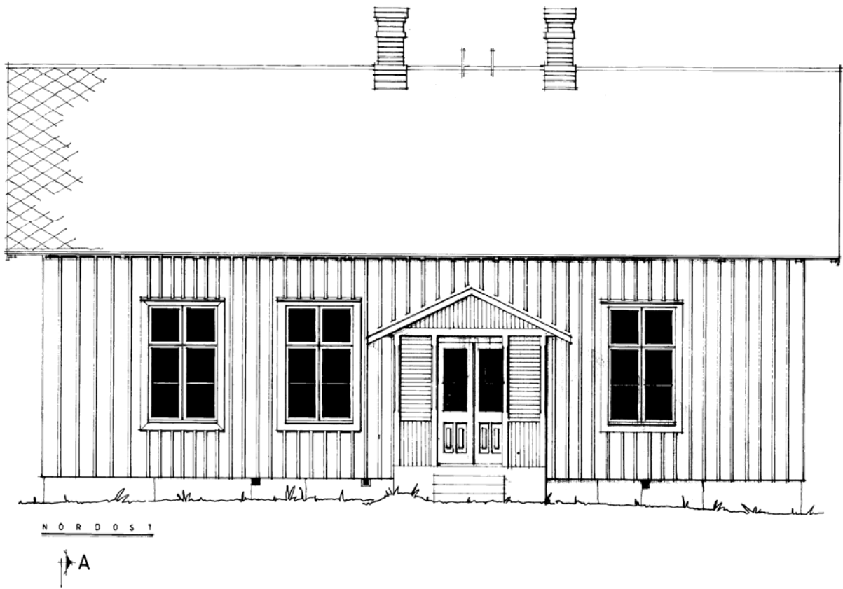
Nordöstra fasaden.
