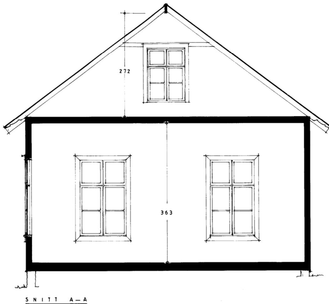
Sektion genom skolsalen.
