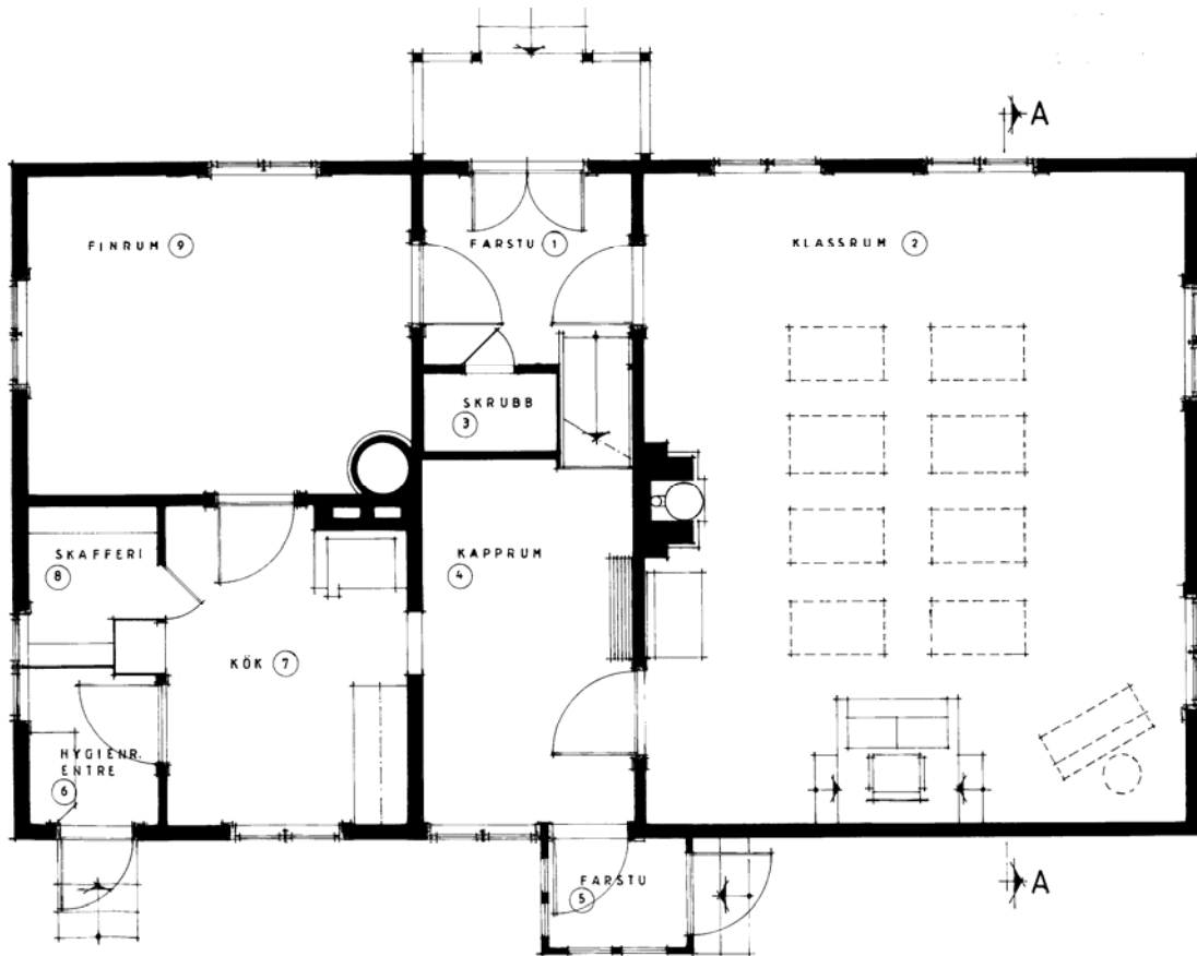
Plan första våningen.
