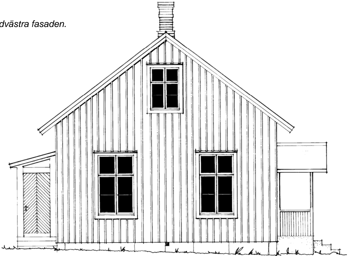
Sydöstra gaveln.
