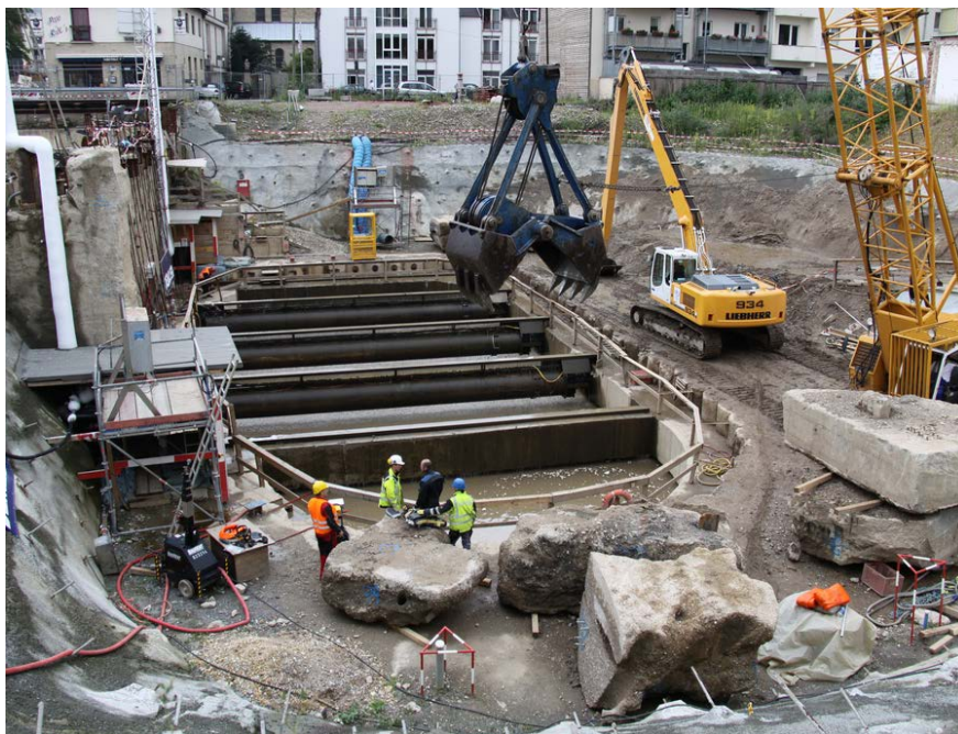
Grundwasserbergung – Bergungsbauwerk
