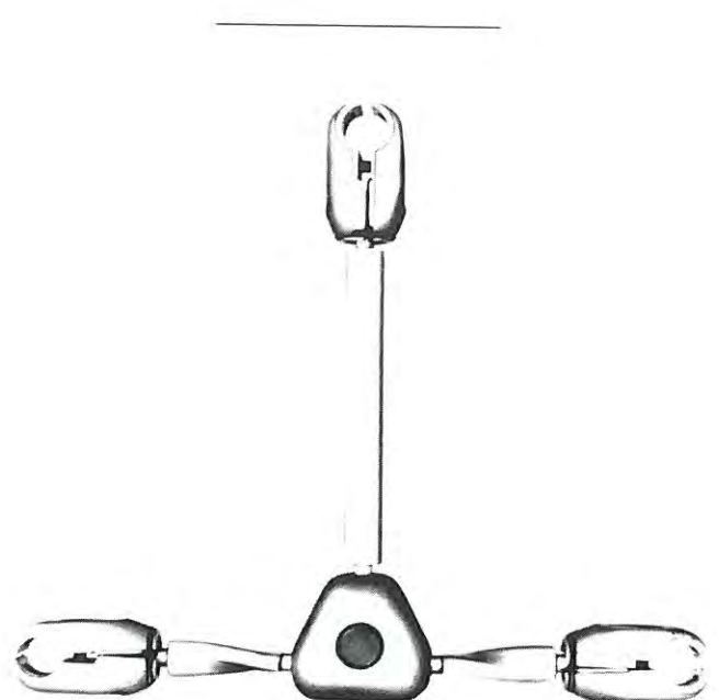
Fig. 6-11. EHV 3/C bundle/phase spacer-damper.
