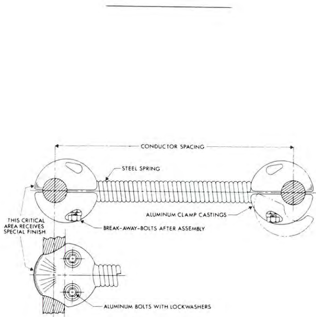
Fig. 6-10. EHV 2/c bundle/phase spacer-damper.
