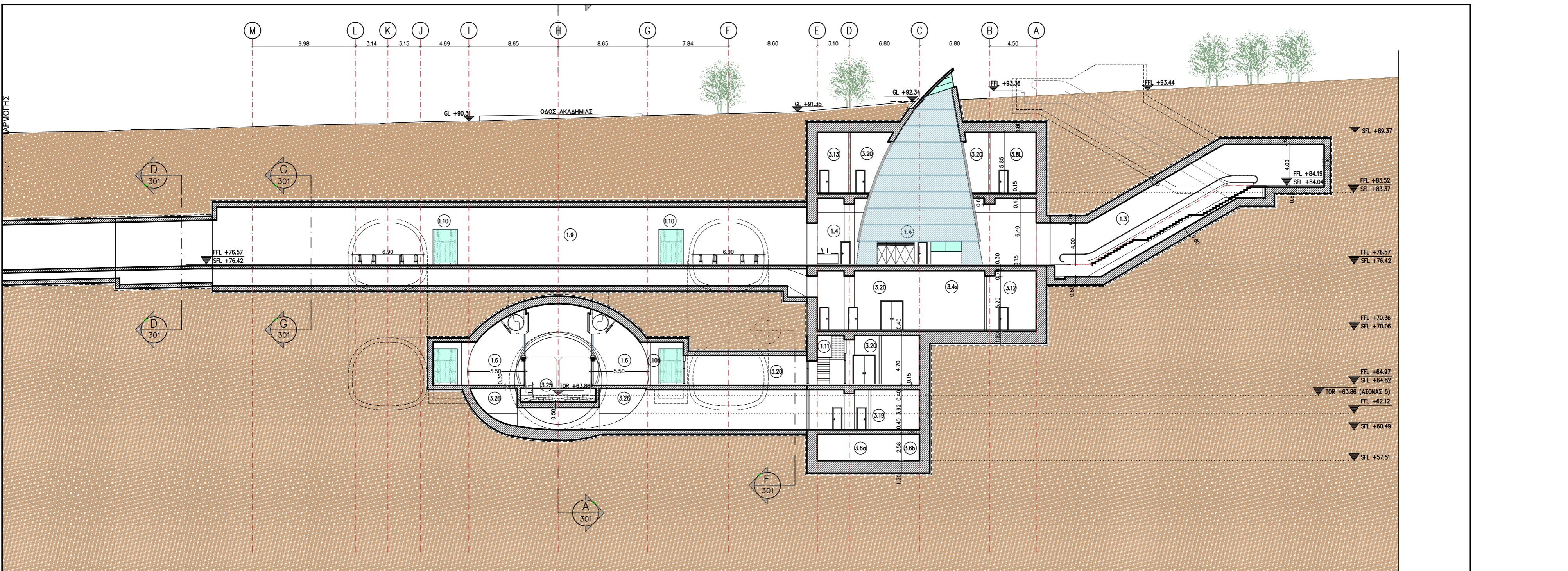
TOMH B-B ΚΛΙΜΑΚΑ 1:200
