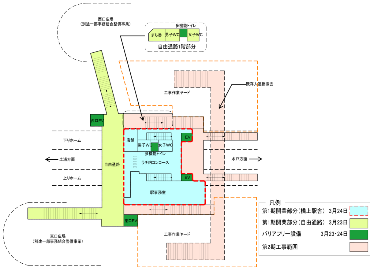
神立橋上駅2階平面
