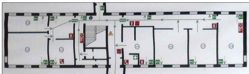
План 1-го этажа (противопожарная схема)
