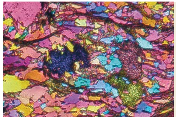
Mikroskooppikuva ohuthiestä.
