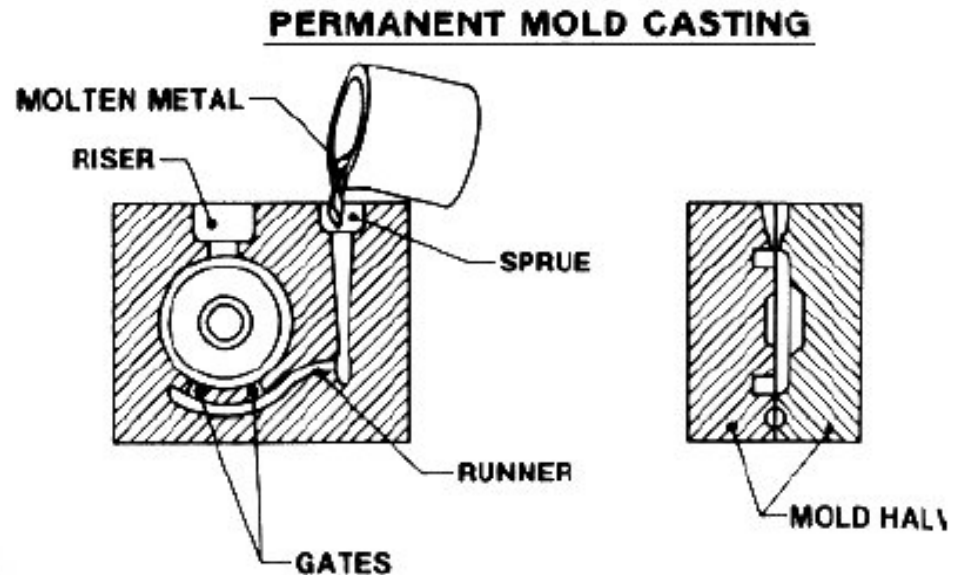
Gravitacijsko lijevanje u kokile
