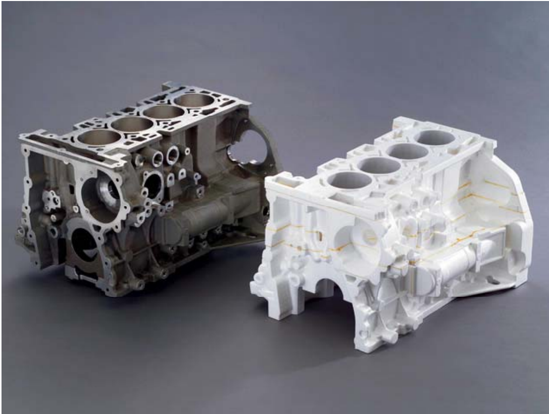
BLOK MOTORA – ODLJEVAK - MODEL
