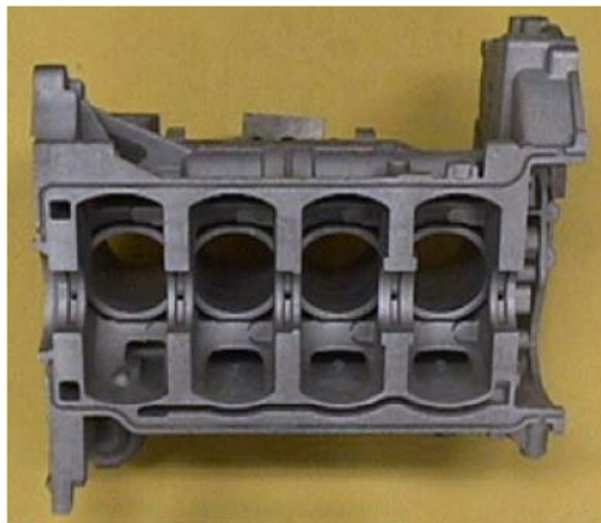
Blok motora
