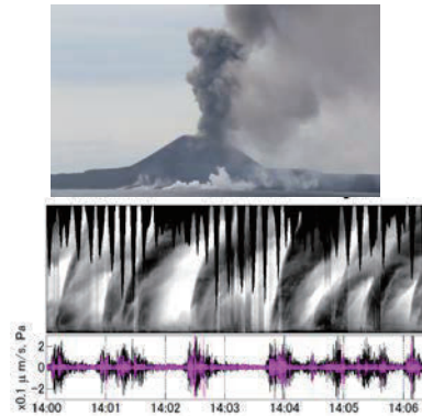
衛星画像、海底地震計、空振計、海洋調査船等を用いた西之島火山の観測
