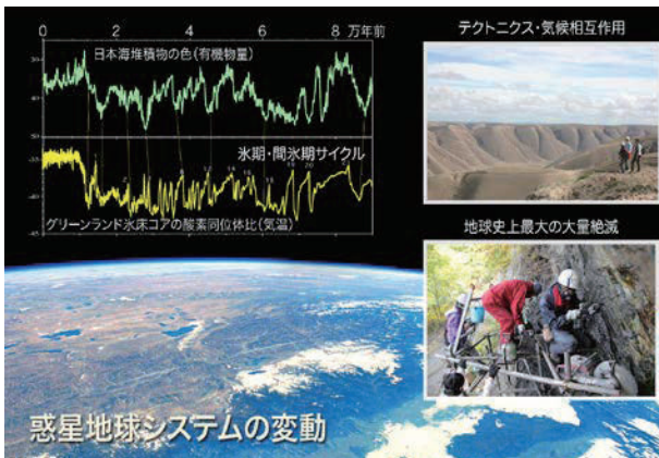
(左) 堆積物の有機物含有量に記憶された数千年規模の急激な気候変動。(右上) テクトニクスと表層環境の相互作用によるモンスーン気候の成立・強化。(右下) 史上最大の大量絶滅
