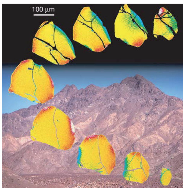
マントル物質の直接観察。鉱物内の元素分布から変形流動過程を知る。
