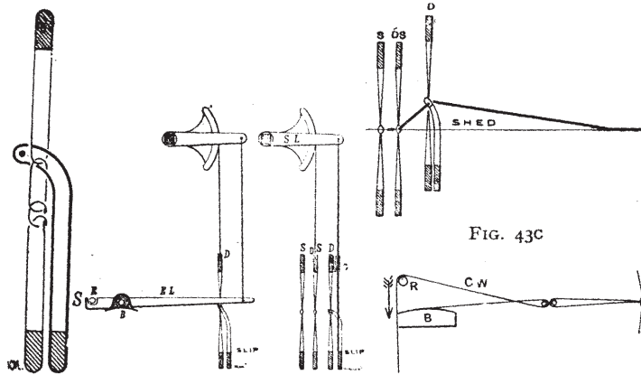
FIG. 42. FIG. 43A. FIG. 43B. FIG. 43C.
