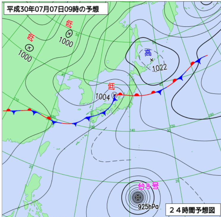
予想天気図 (7月7日9時予想)
