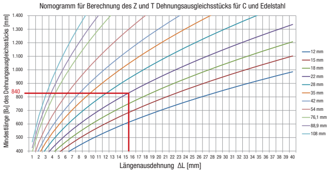
GRAFIK 1: NOMOGRAMM (FÜR EDELSTAHL) FÜR DIE BERECHNUNG DER SITUATION ABBILDUNGEN 13 UND 14 DEHNUNG B_d [mm]
