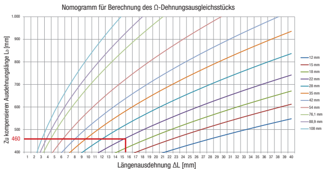
GRAFIK 2: NOMOGRAMM FÜR DIE BERECHNUNG DER SITUATION ABBILDUNG 15 DEHNUNGS-AUSGLEICHSTÜCKS L_b [mm]
