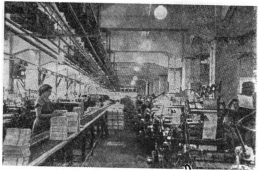
Потоково-механізована лінія для виготовлення книг на книжковій фабриці імені М. В. Фрунзе. Харків.
