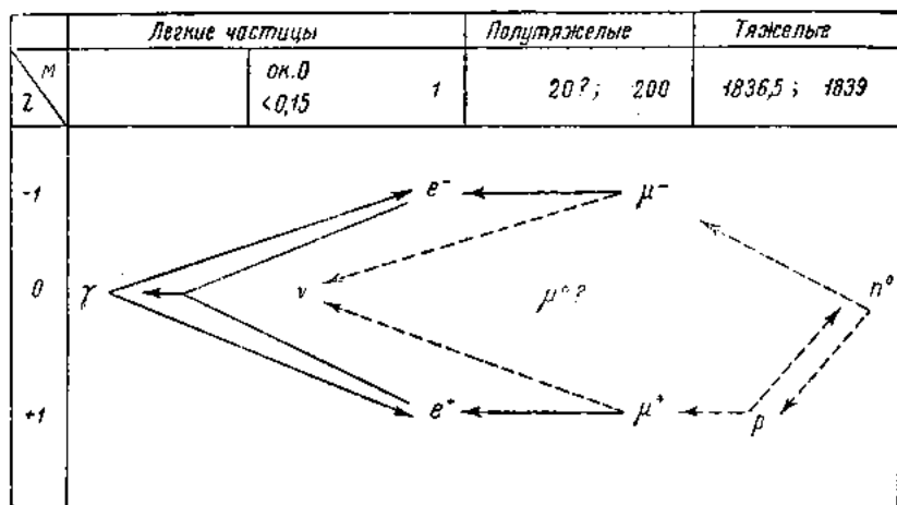
Схема эволюции «элементарных» частиц (1941 г.)
