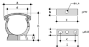
Clip
