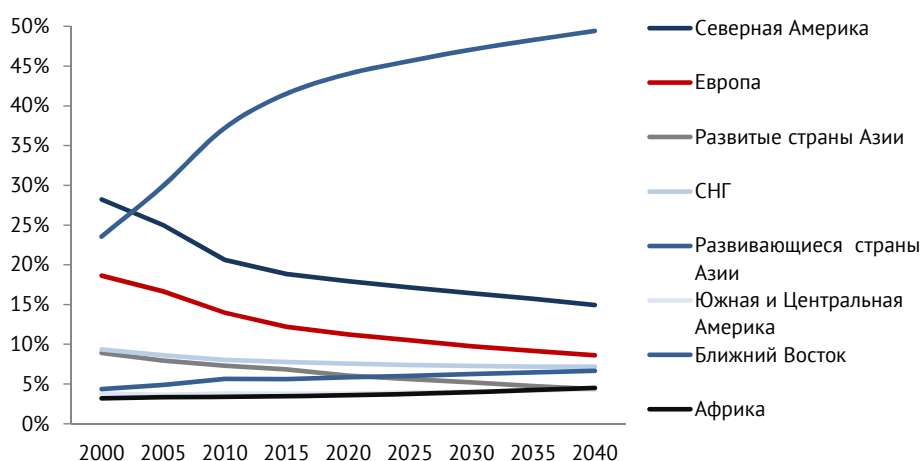
Рисунок 1.78 – Выбросы по регионам (процент от мирового)
