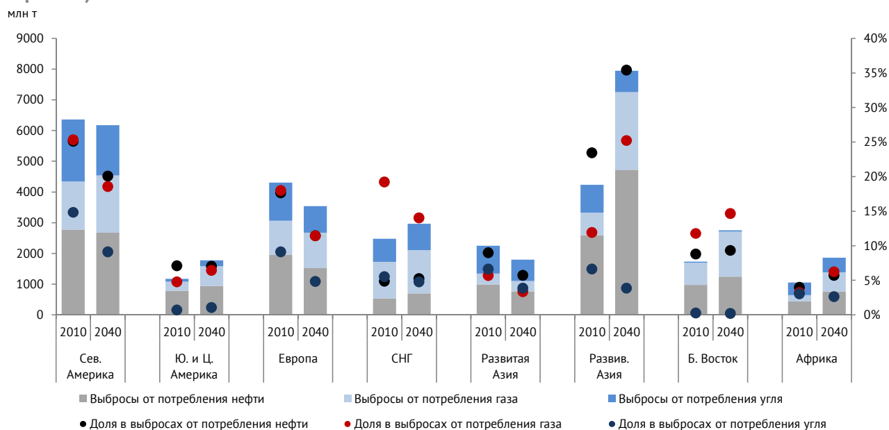
Рисунок 1.79 – Структура выбросов по регионам по видам топлива (абсолютный объем и процент от мирового)
