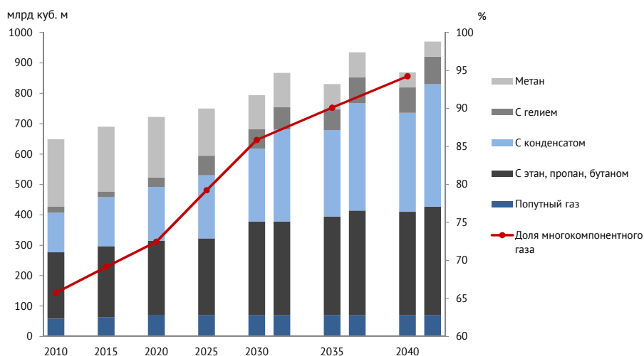
Рисунок 3.31 – Состав добываемых газов
