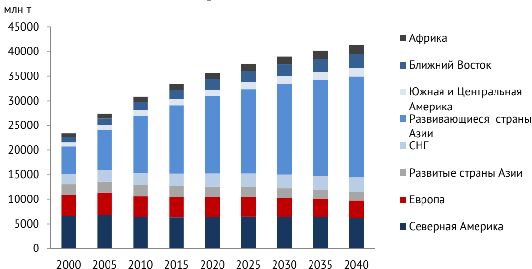
Рисунок 1.77 – Динамика выбросов CO 2 по регионам
