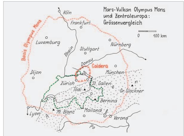
In die Kartenskizze der Schweiz und Umgebung sind massstäblich korrekt die Umrisse und die Caldera von Olympus Mons rot eingezeichnet.
