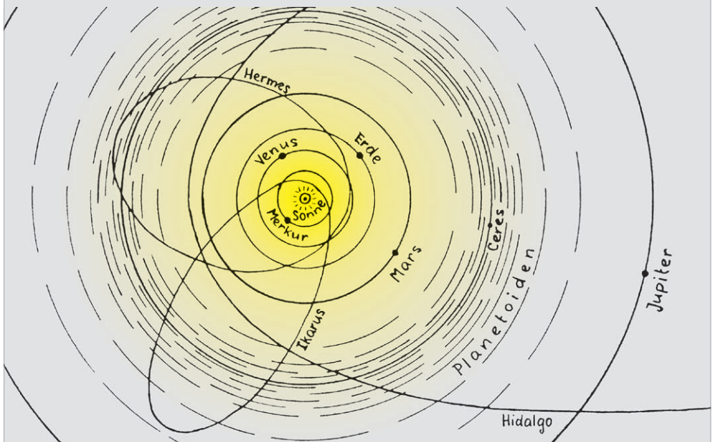
Planetoiden-Bahnen mit Sonderfällen (massstäblich)
