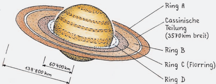
Ansicht des Saturn
