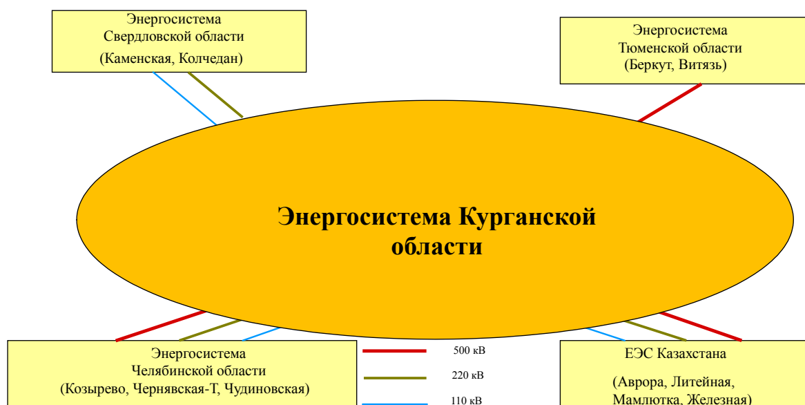
Рисунок 3. Внешние связи энергосистемы Курганской области
