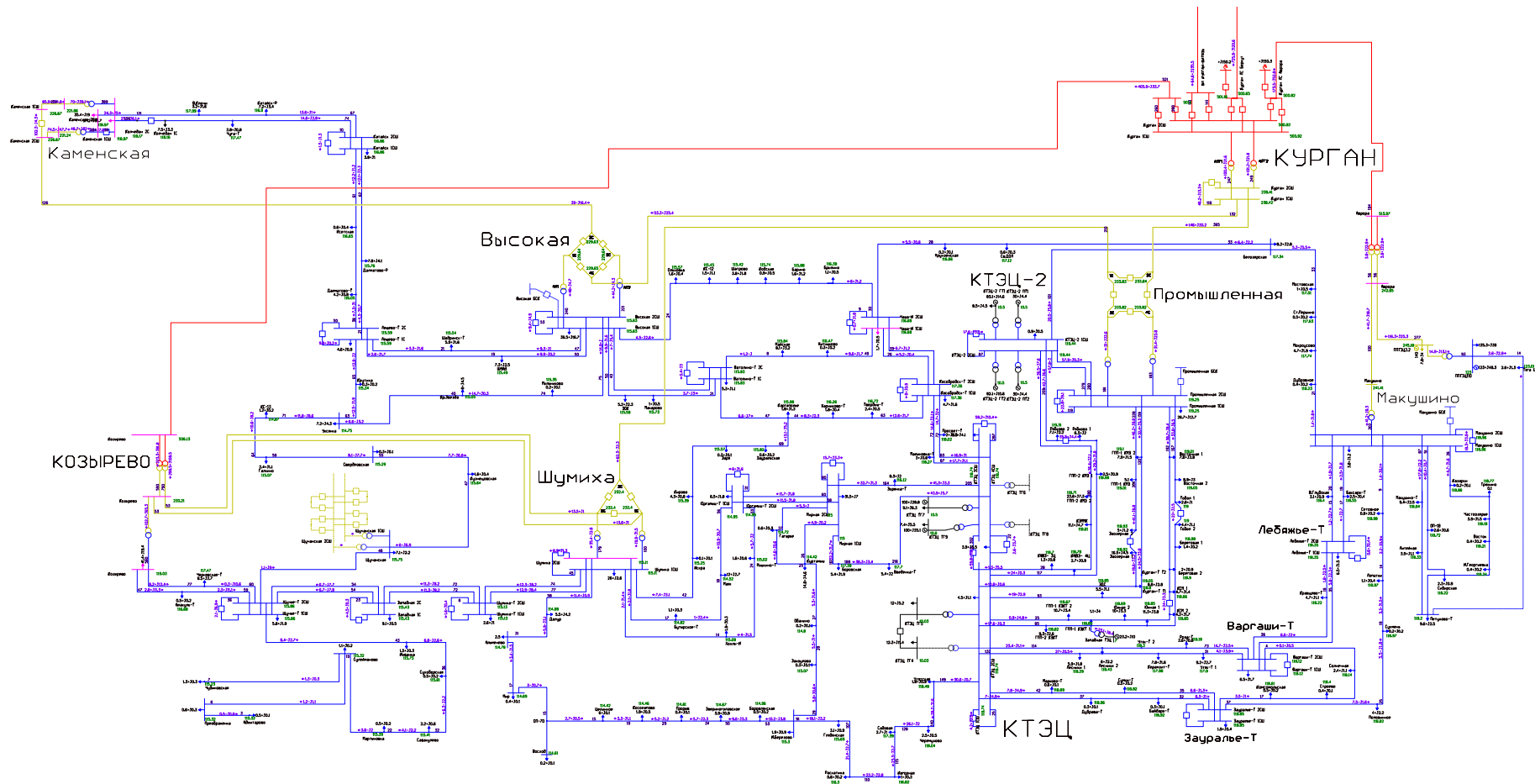
Рисунок 7. Режим зимних максимальных нагрузок рабочего дня энергосистемы Курганской области (2023 г.)
