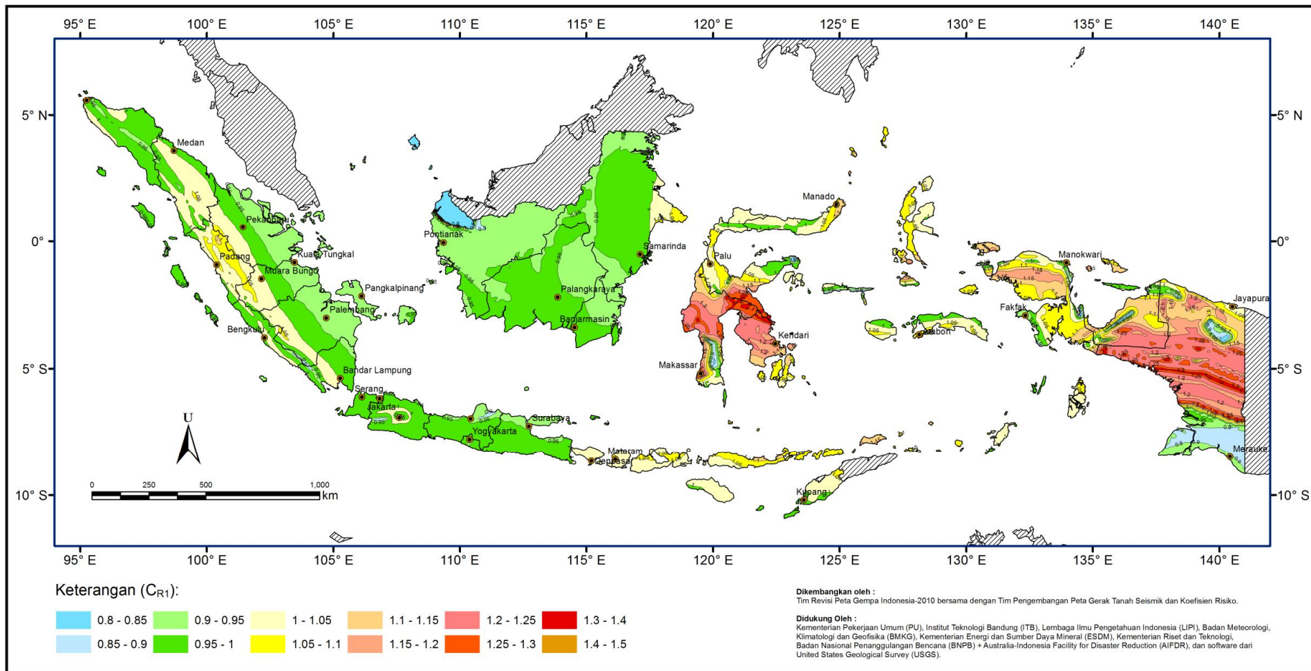
Gambar13 - C_{R1} , Koefisien risiko terpetakan, periode respons spektral 1 detik
