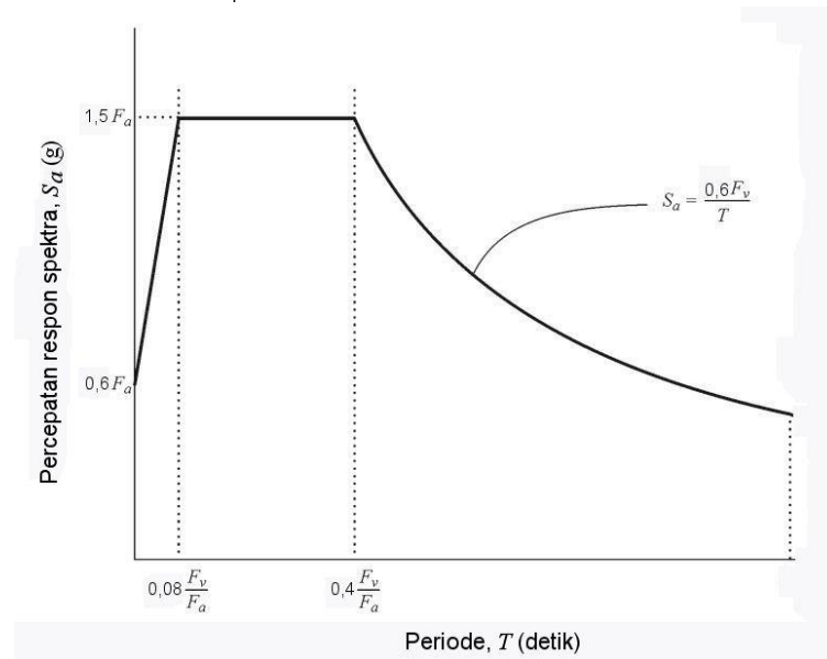
Gambar 2 - Batas Bawah Spektrum Respons MCE_R Deterministik
