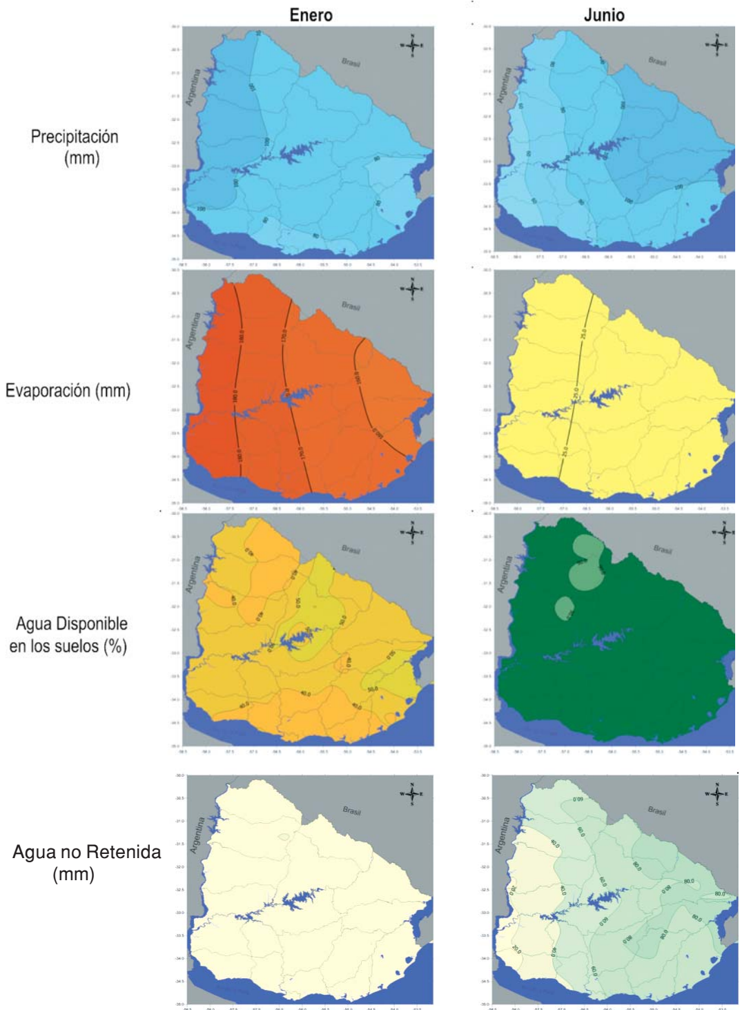
Figura 19. Precipitaciones, evaporación, porcentaje agua disponible y agua no retenida mensual promedio de los meses de enero y junio (mediana 1985-2009).
