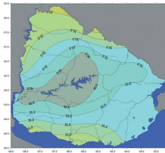
Figura 15. Días con heladas acumulado anualmente meses mayo-octubre (mediana 1980-2009)
