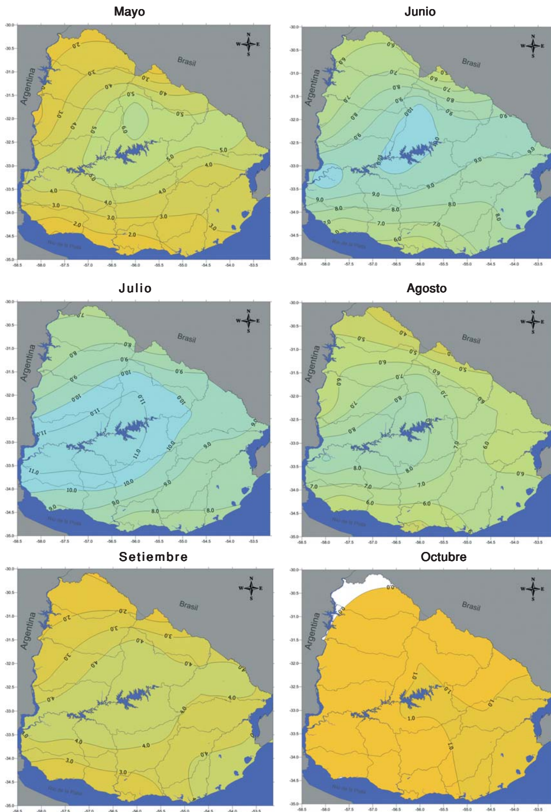
Figura 16. Días con Helada acumulado mensual (mediana 1980-2009).
