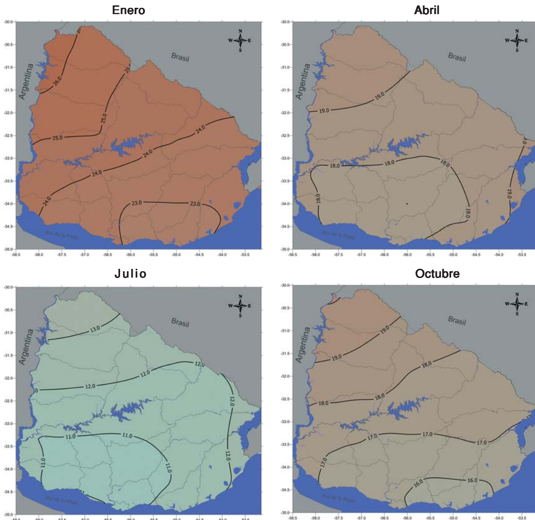
Figura 4. Temperaturas medias mensuales (°C) en enero, abril, julio y octubre (mediana 1980-2009).
