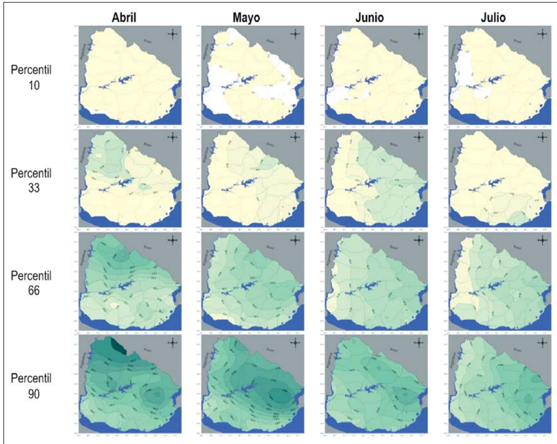
Figura 26. Percentiles de agua no retenida por los suelos mensual (mm) en abril, mayo, junio y julio (1985 – 2009).
