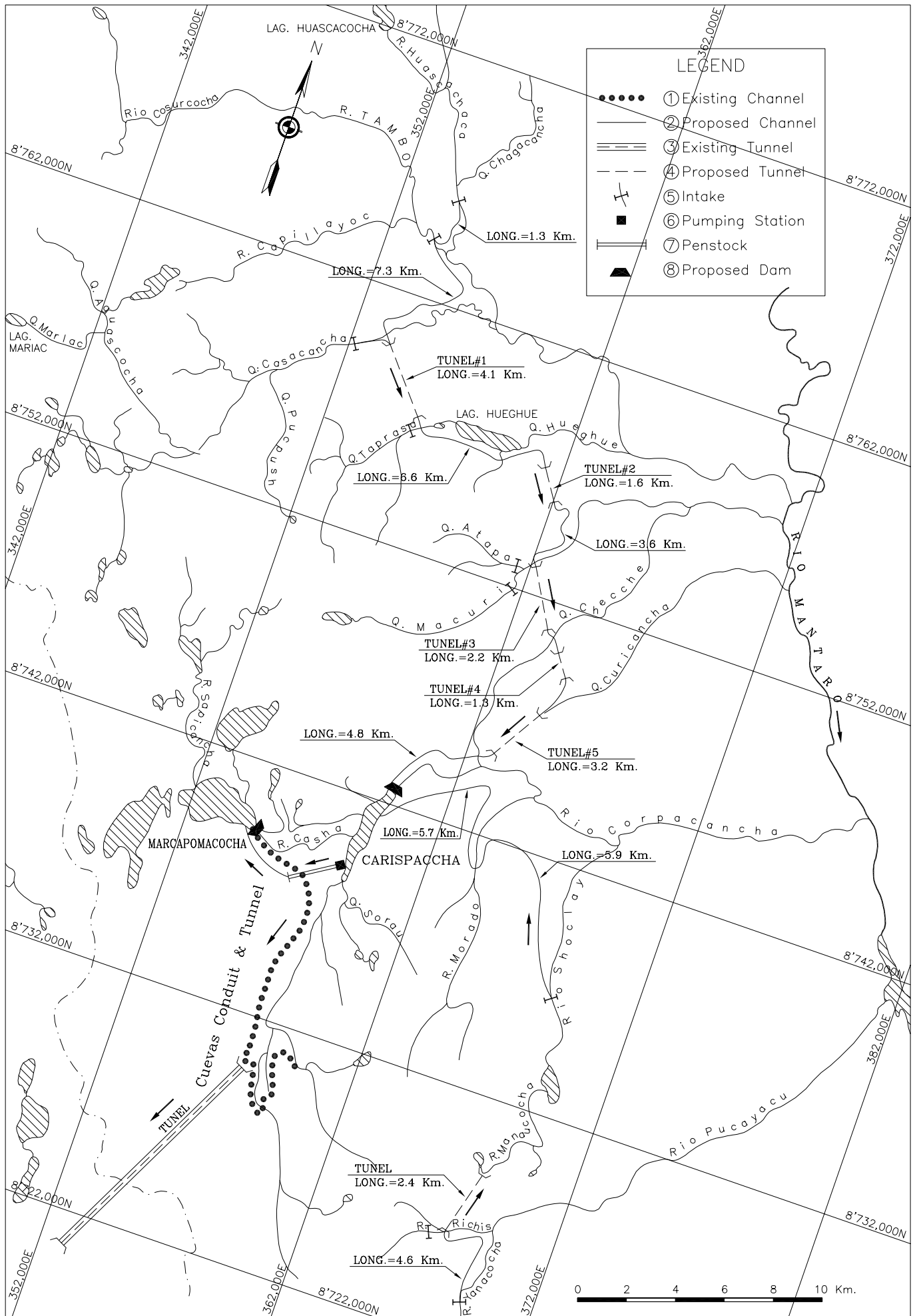
Figura 5.1.10 Planta General de Conduccion de Agua del MANTARO (Etapa-1 y Etapa-2)
